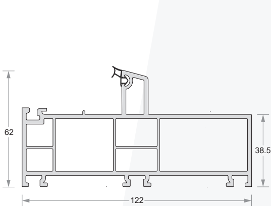
Casement Twin Villa Frame Code- DP67-ET-775
