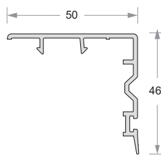
Sliding Door Interlock Code- DP67-ET-711
